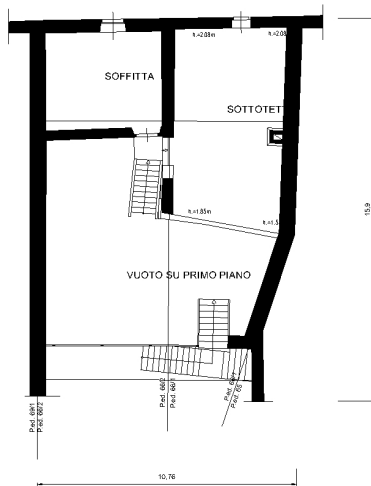
Piano secondo (sottotetto)
