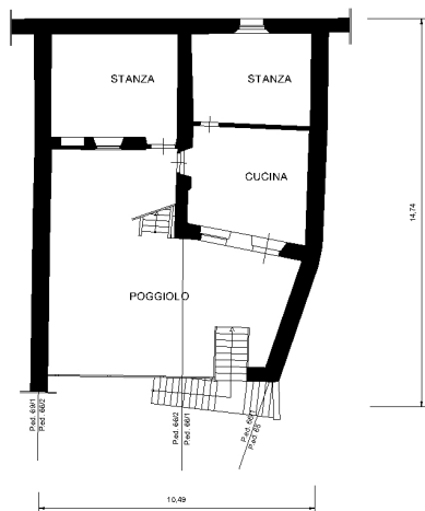
Piano primo
